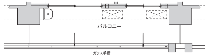
7~8階バルコニー
