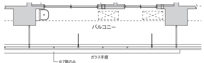
7～8階バルコニー
