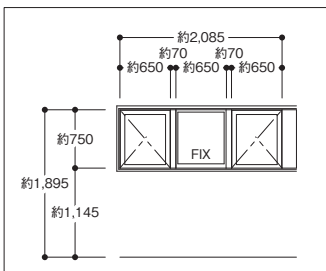
LDコーナー 窓姿図 東側
