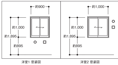
洋室1 窓姿図
