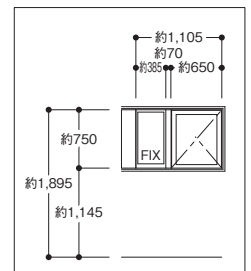
LDコーナー 窓姿図 南側
